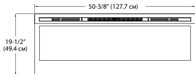
ФРОНТАЛЬНАЯ СТОРОНА
